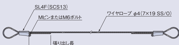
標準仕様 組立例 (mm)
