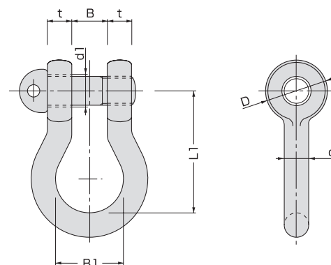
■寸法図
