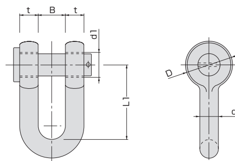
■寸法図
