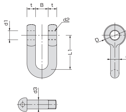
■寸法図
