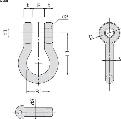
■寸法図
