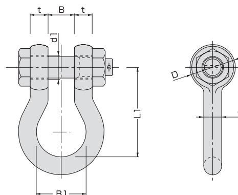
■寸法図
