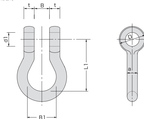
■寸法図
