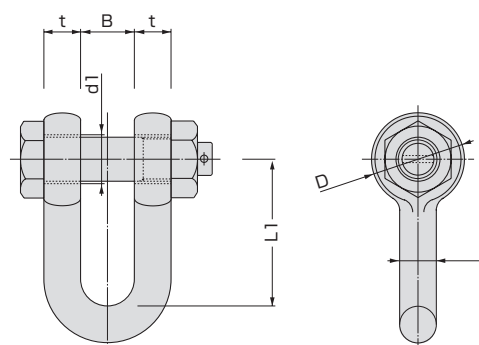
■寸法図
