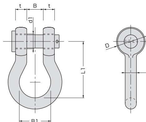
■寸法図
