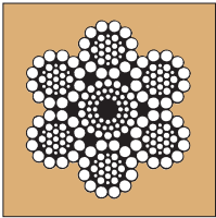
ロータレスロープ SeS (48) + 6 × WS (31)
