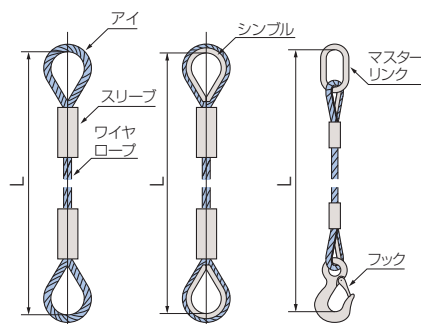
図1●1本形の例
