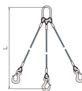
図3●3本形の例
