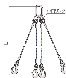
図4●4本形の例
