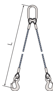
図2●2本形の例
